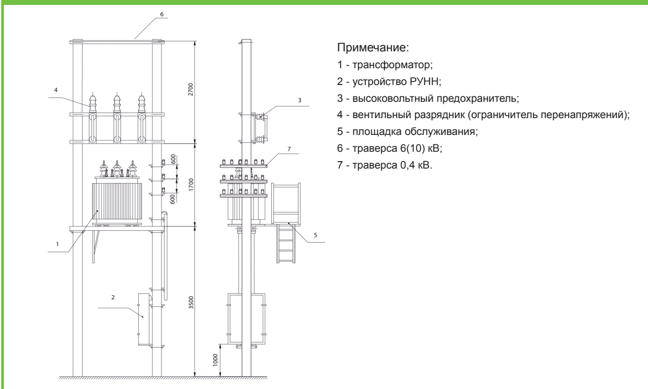
Рисунок 2.1 Общий вид и габаритные размеры МТП
