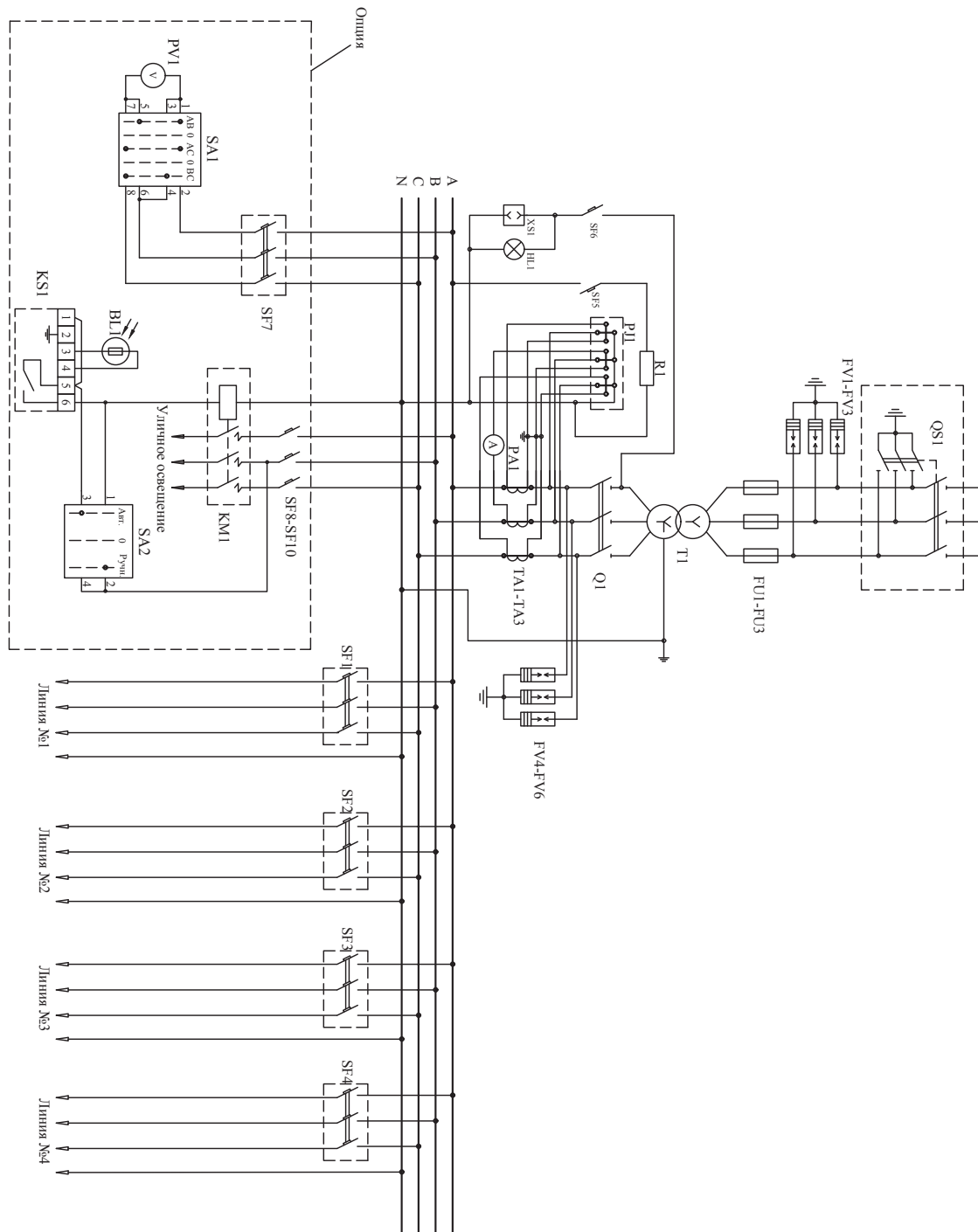
Рисунок 4.2 Схема электрическая принципиальная КТПс
