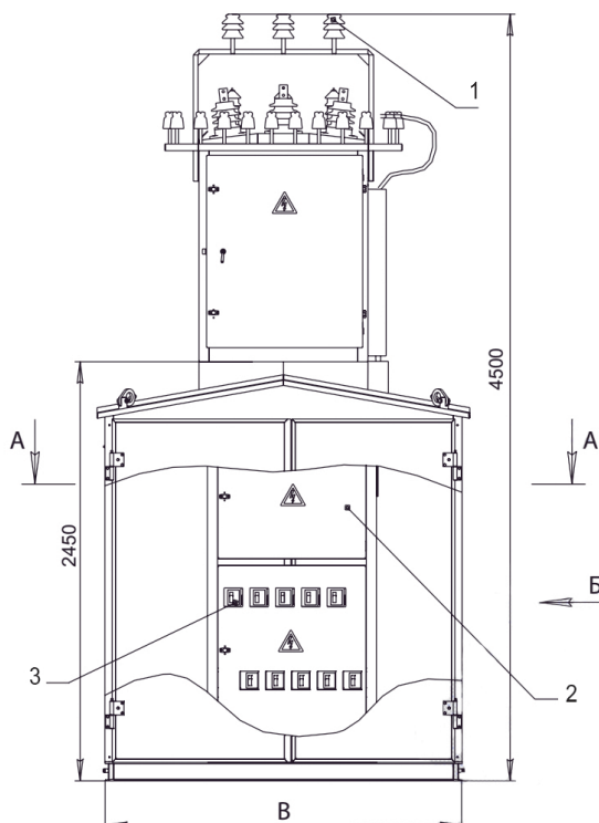
Рисунок 3.1 Общий вид и габаритные размеры КТПН
