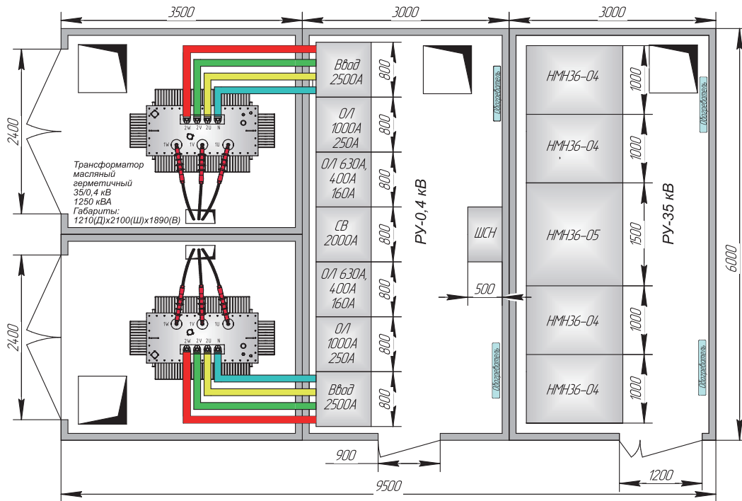
Рисунок 9.2 Схема электрическая принципиальная КТПМБ
